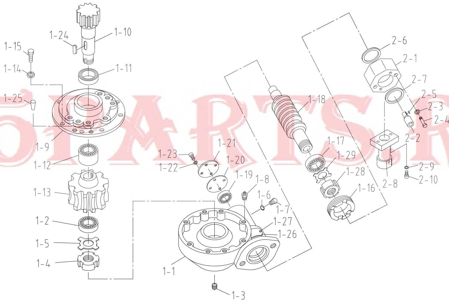
스윙 감속기 조립체 Fig. 3-1 SCS746L SWING R/G ASS'Y
