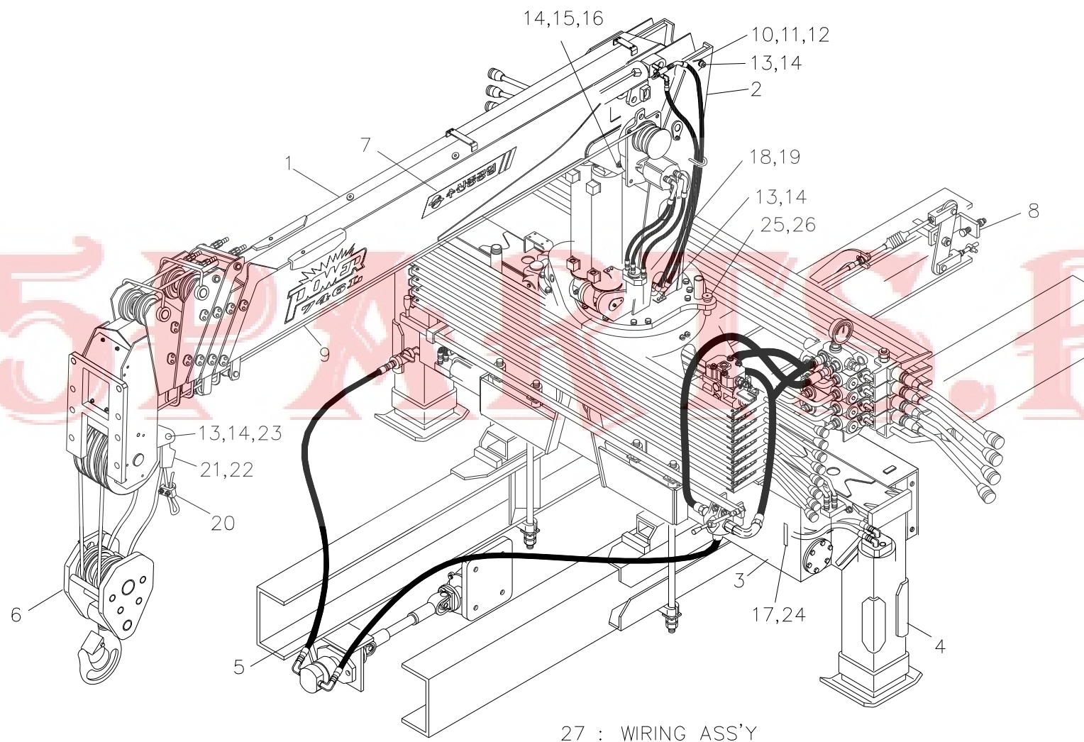
크레인 조립체 (표준형) Fig. 0 SCS746L CRANE ASS'Y (STD)
