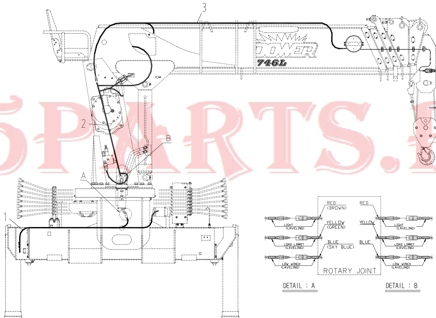
전선 조립체 Fig. 10 SCS746L WIRING ASS'Y (TOP)
