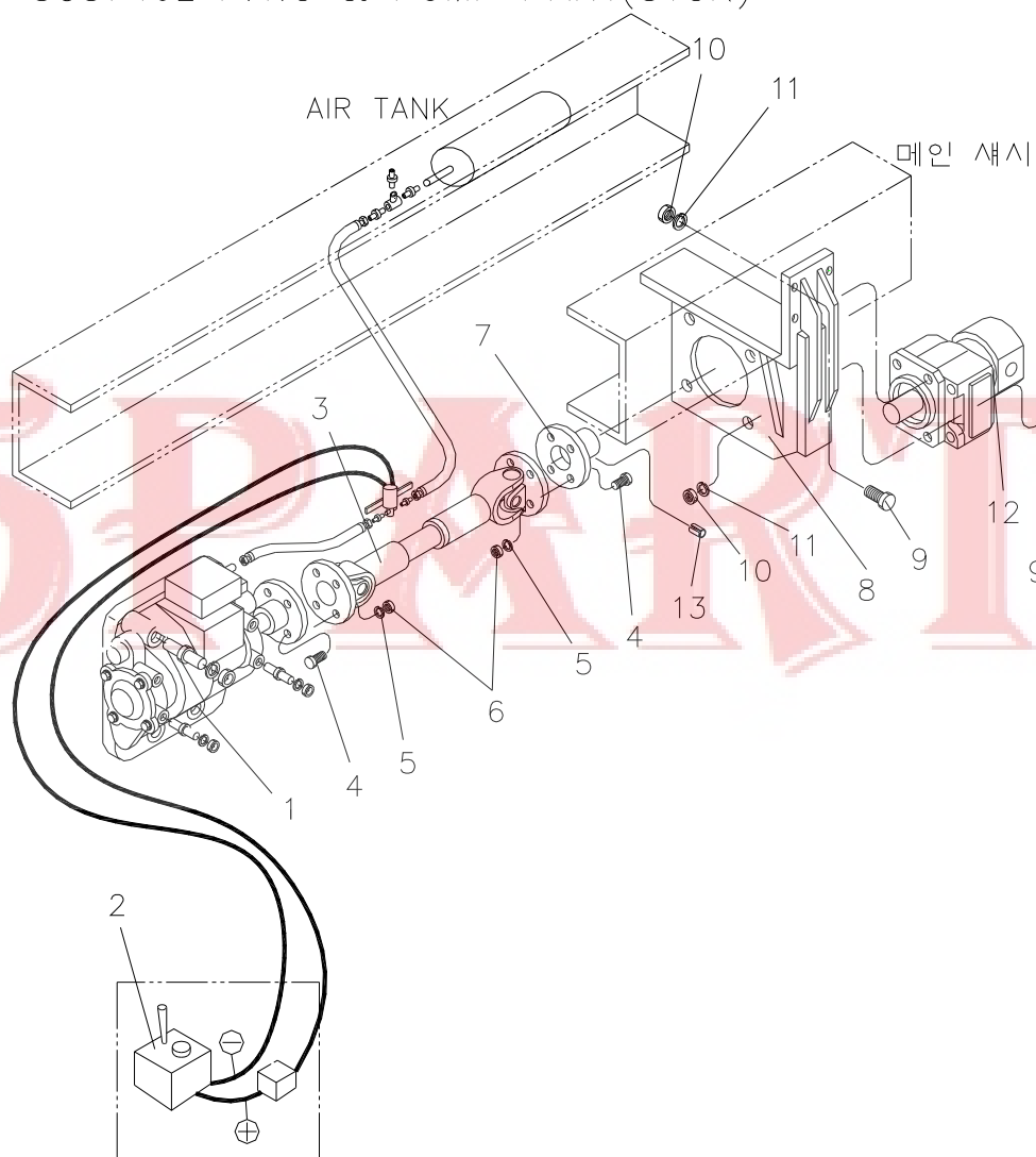
동력인출장치 & 펌프파트(8톤) Fig. 8-1 SCS746L P.T.O & PUMP PART(8TON)
