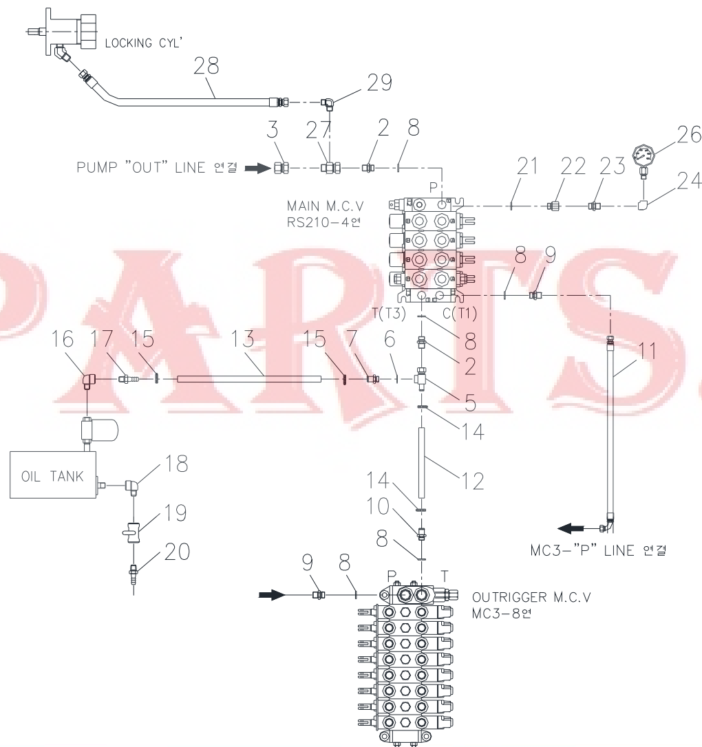
디스트리뷰터 배관 (표준형) Fig. 5-1 SCS746L DISTRIBUTOR PIPING (STD)
