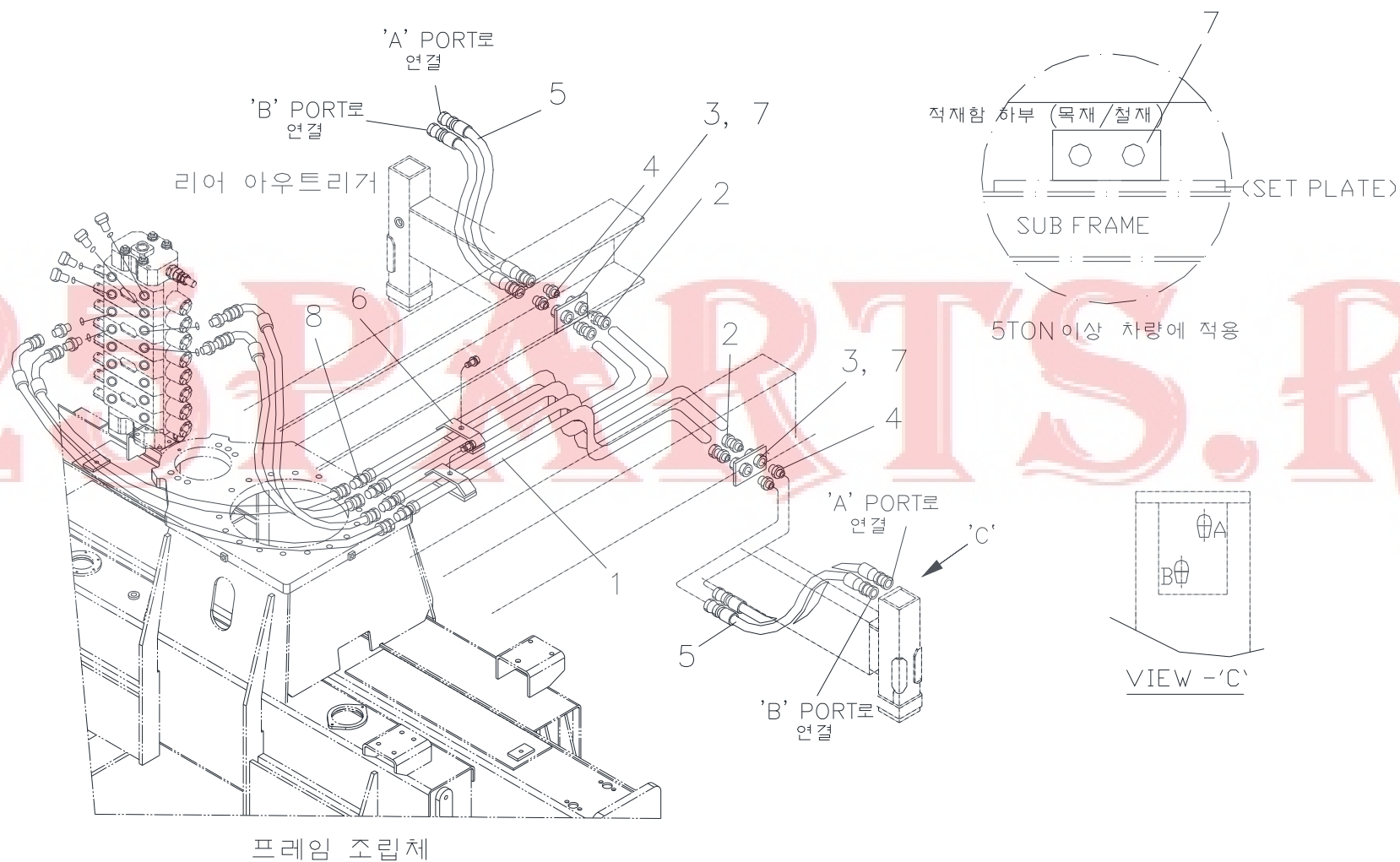
후방 장착 배관 파트 Fig. 8-4 SCS514 R/O M/T PIPING PART
