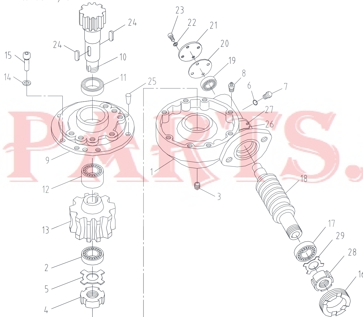
스윙 감속기 셋트 Fig. 3-1 SCS514 SWING R/G SET
