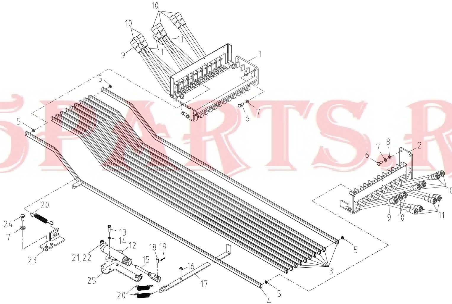
오퍼레이션 조립체 Fig. 3-2 SCS1616 OPERATION ASS'Y
