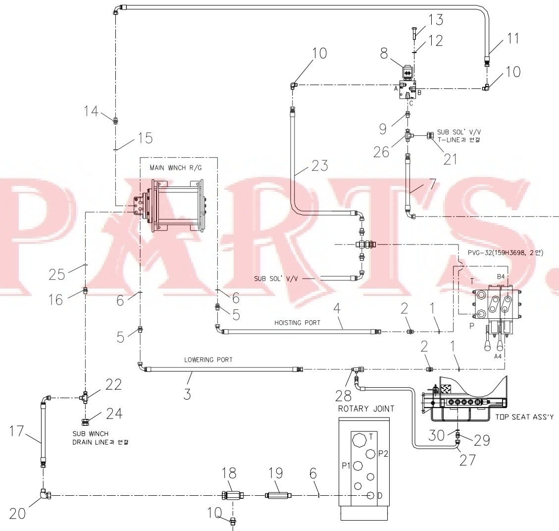
메인 윈치 배관 Fig. 5-5 SCS1616 MAIN WINCH PIPING
