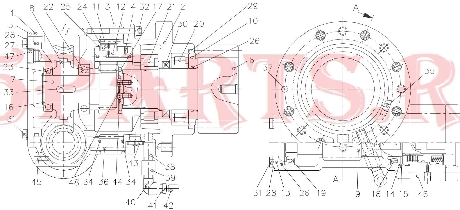
SECTION A-A
