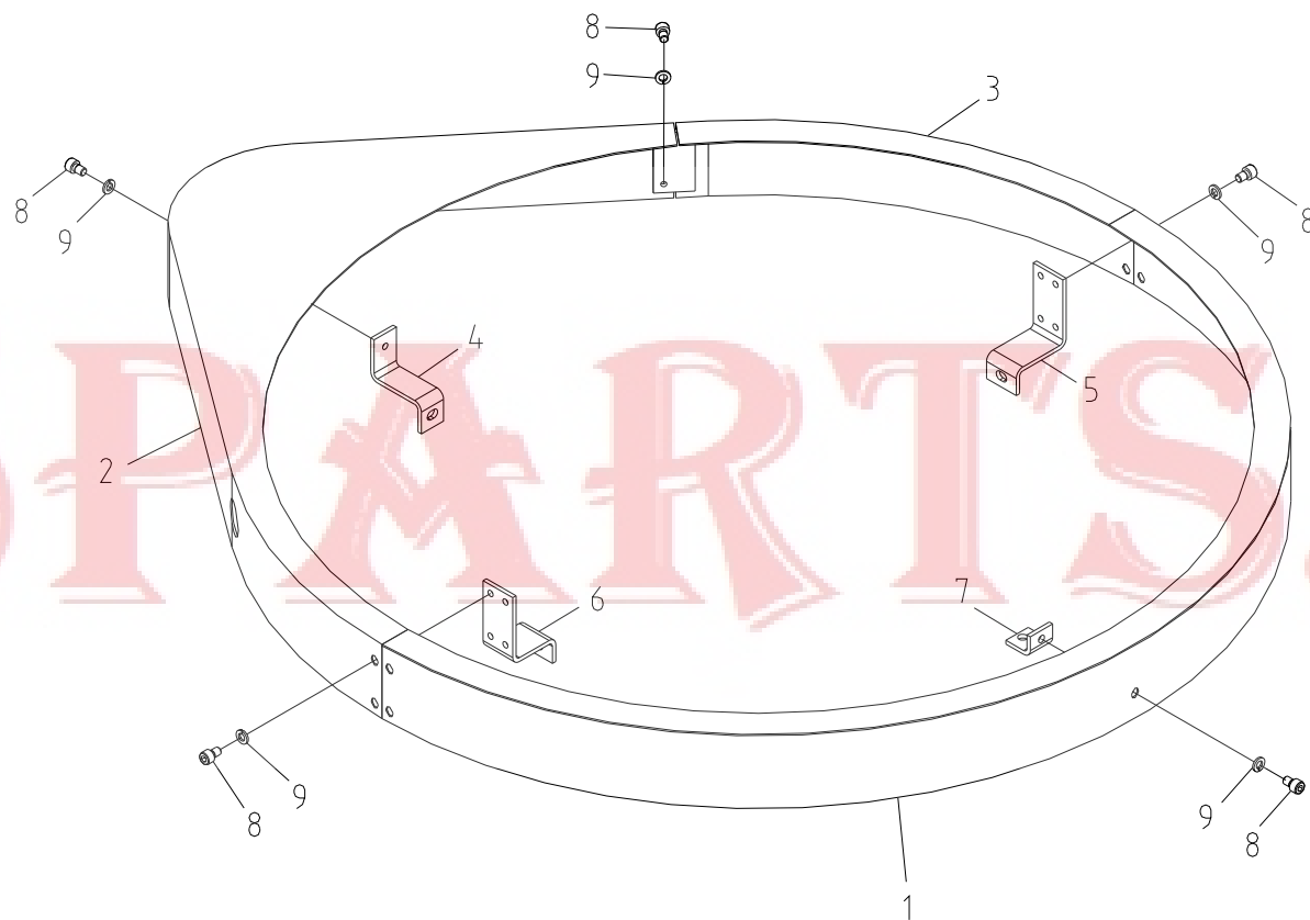
기어 커버 세트 Fig. 3-3 SCS1616 GEAR COVER SET
