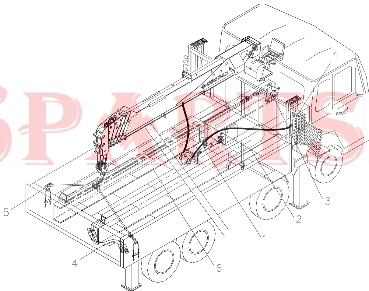
장착 조립체 Fig. 9 SCS1616 MOUNTING ASS'Y
