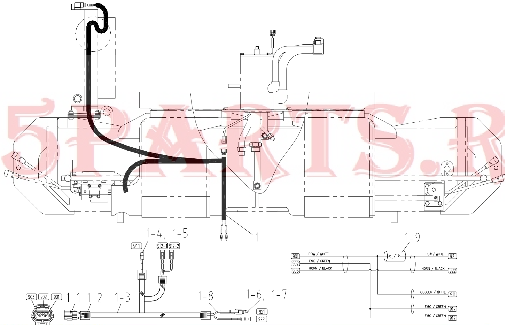
프레임 전선 Fig. 11-1. SCS1015LS FRAME WIRING
